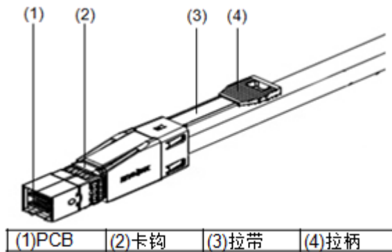
图4-33 SAS 线缆上 Mini SAS HD 连接器示意图
