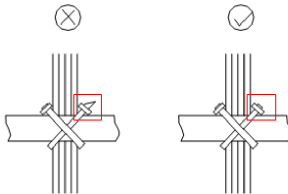
图4-21 线缆捆扎示意图（二）
