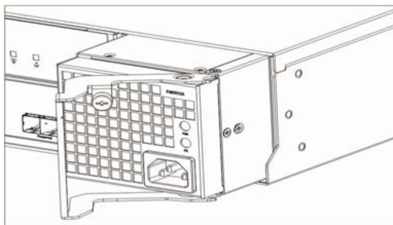
图4-18 安装 DSU5625B 风扇模块+电池模块+电源模块示意图
