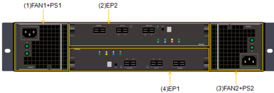
图3-29 DSU5625 后正视图
