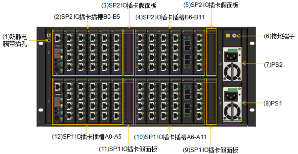
图3-3 SPU 后正视图
