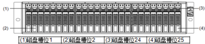
图6-18 DSU 磁盘槽位编号示意图（一）
