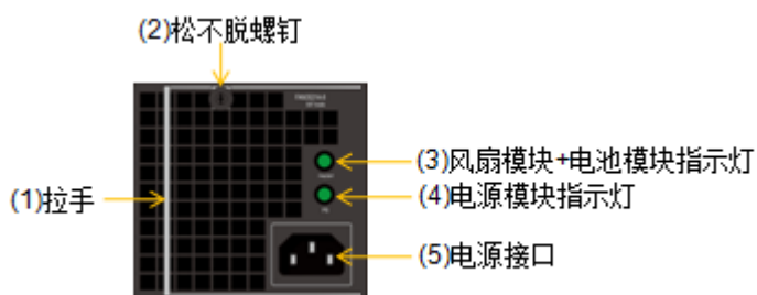
图3-31 DSU5625B 风扇模块+电池模块+电源模块正视图
