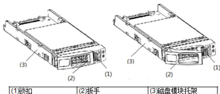
图6-17 2.5 英寸磁盘模块示意图
