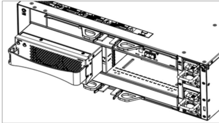
图6-10 安装/拆卸 DSU2624B 风扇模块+电池模块示意图
