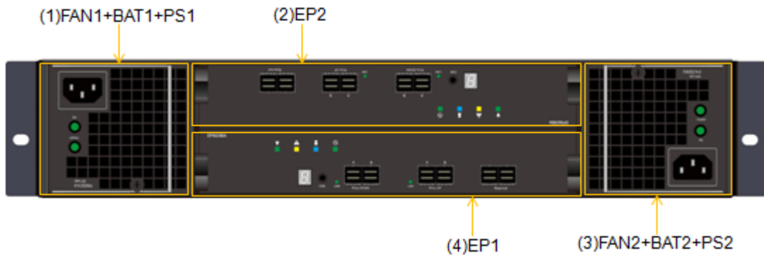
图3-28 DSU5625B 后正视图
