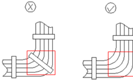
图4-22 线缆捆扎示意图（三）
