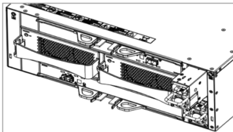
图6-16 安装/拆卸 DSU2624 电源模块示意图
