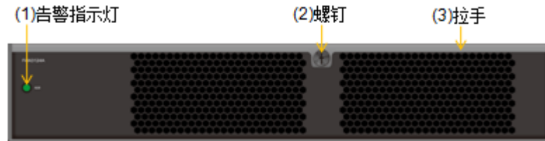
图3-6 SPU 风扇模块正视图
