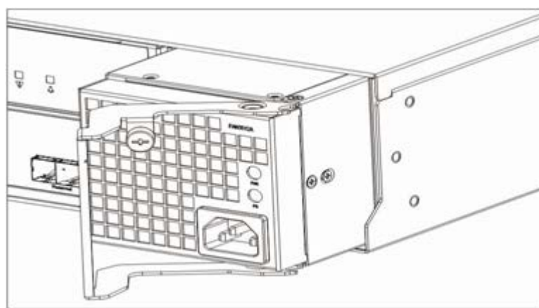
图6-15 安装/拆卸 DSU5625 风扇模块+电源模块示意图
