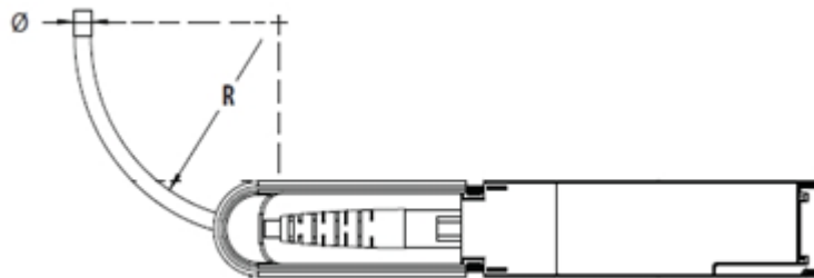
图4-35 AOC 光缆弯曲半径示意图
