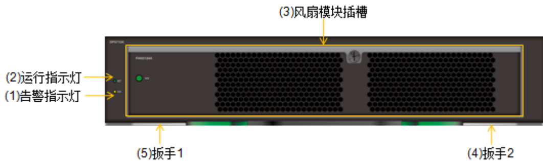
图3-4 SP 正视图
