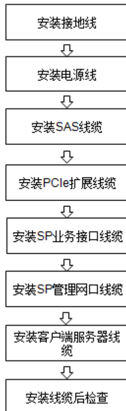
图4-23 线缆安装流程示意图
