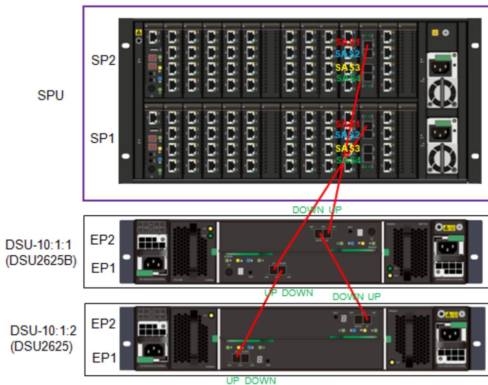
图4-36 SAS1 接口上 SAS 线缆安装示意图
