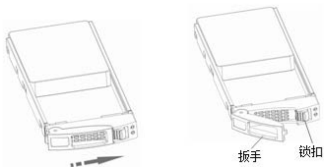
图6-27 NVMe 磁盘模块示意图
