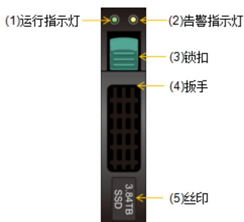
图3-33 NVMe 磁盘模块前面板
