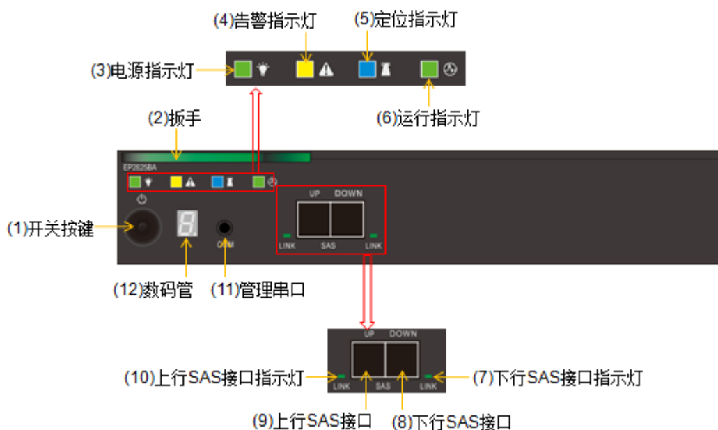
图3-12 DSU2625B 的 EP 正视图
