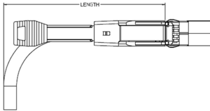
图4-34 铜缆弯曲半径示意图
