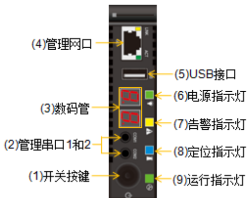
图3-5 SP 管理插卡正视图
