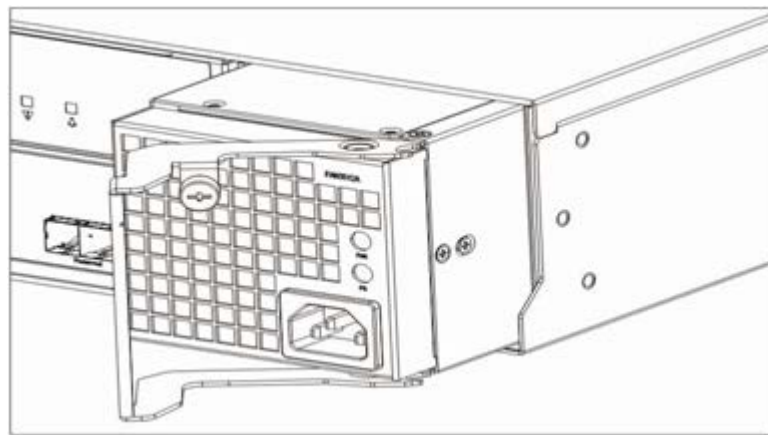
图6-13 安装/拆卸 DSU5625B 风扇模块+电池模块+电源模块示意图
