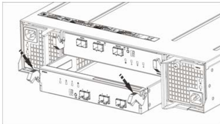
图6-8 安装/拆卸 DSU5625 EP 示意图
