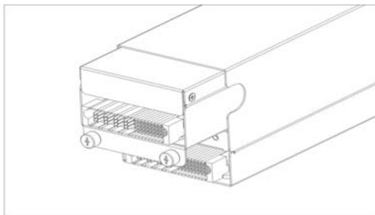
图6-14 安装/拆卸电池模块示意图
