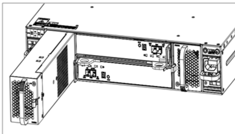
图6-9 安装/拆卸 DSU2625B 风扇模块+电池模块示意图
