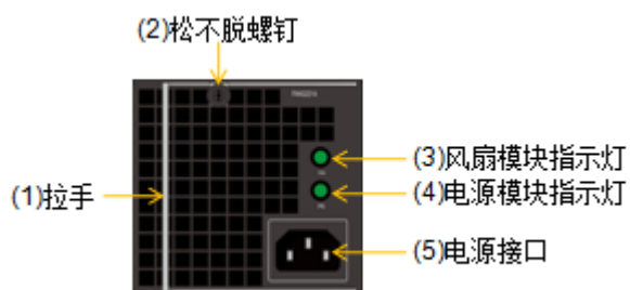
图3-32 DSU5625 风扇模块+电源模块正视图
