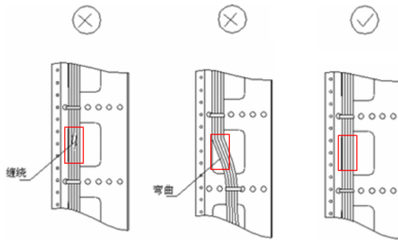
图4-20 线缆捆扎示意图（一）
