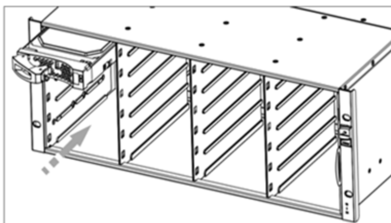
图6-24 安装 3.5 英寸磁盘模块示意图
