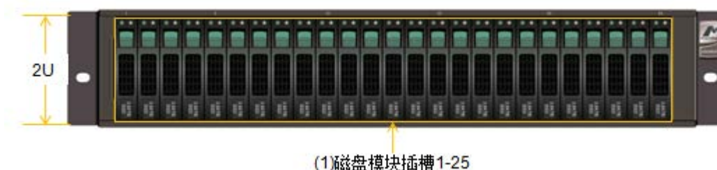
图3-27 DSU5625B/DSU5625 前正视图
