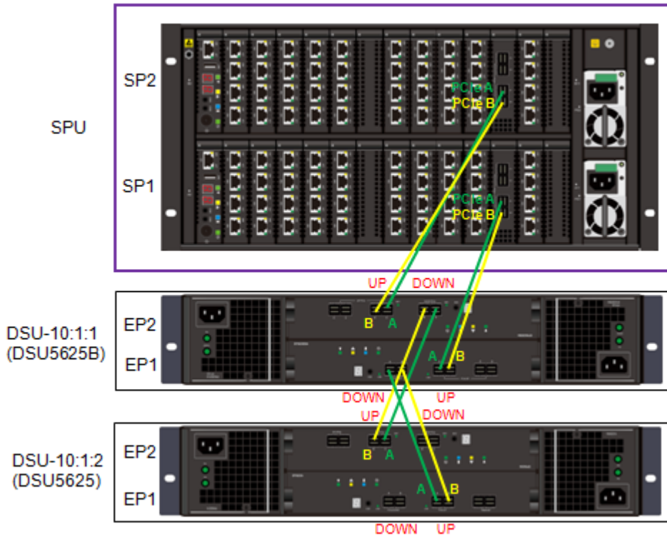
图4-38 PCIe 扩展线缆安装示意图
