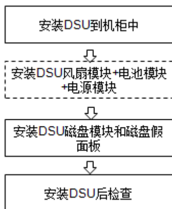
图4-16 DSU 安装流程示意图
