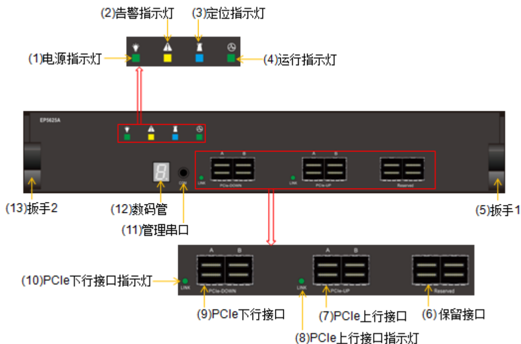
图3-30 DSU5625B/DSU5625 的 EP 正视图
